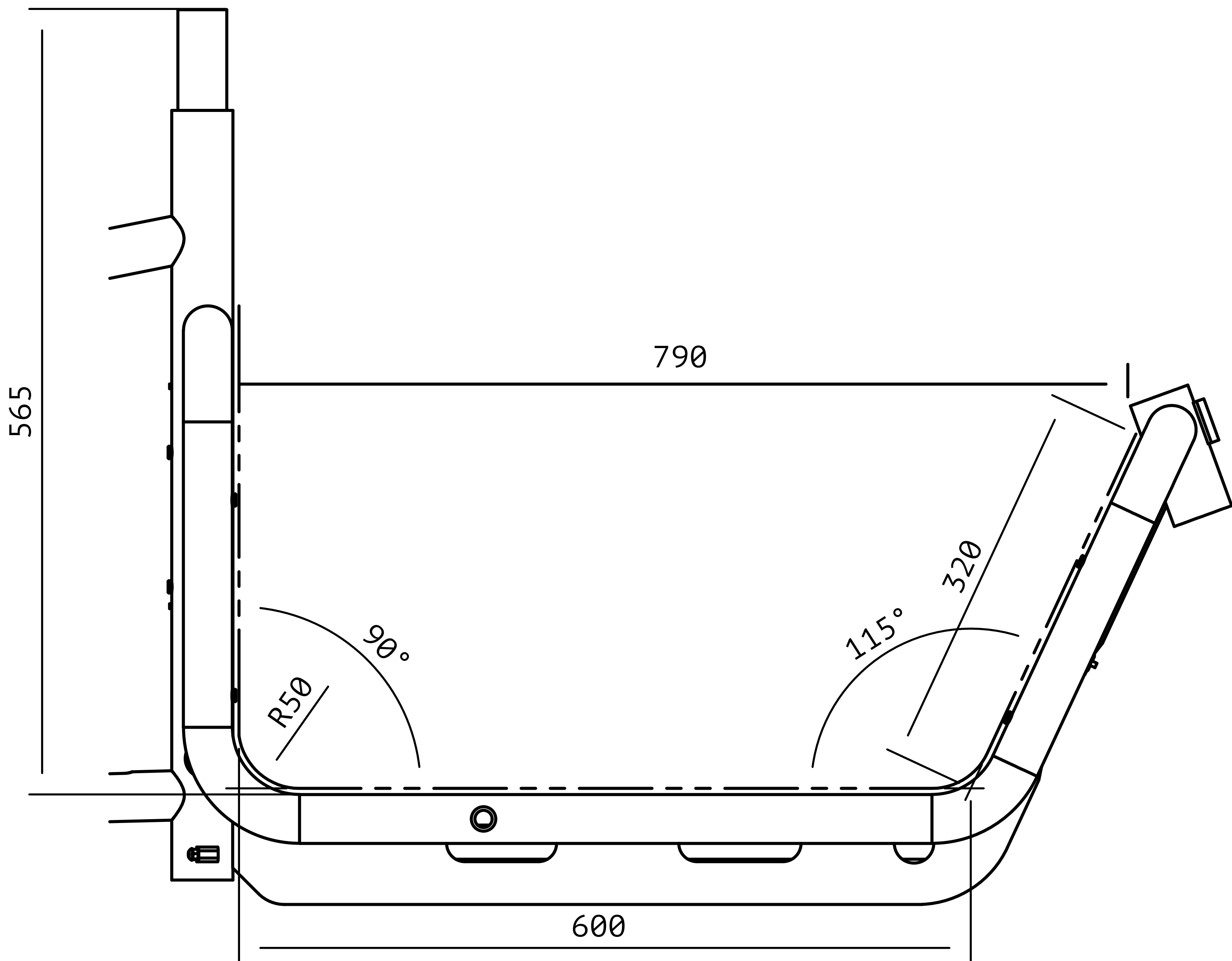
ALLGEMEINE DIMENSIONEN DER LADEFLÄCHE
