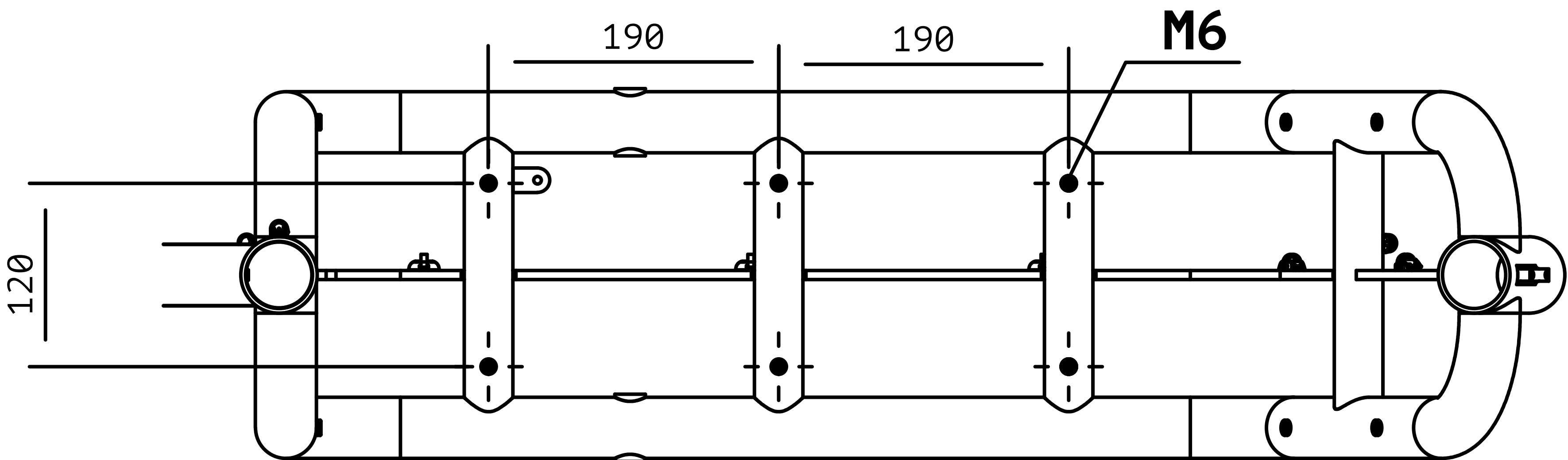
ANSCHRAUBPUNKTE (BODEN)
